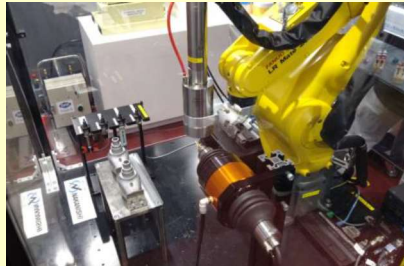
FANUC：バリ取り用ツールチェンジャー付き ロボットシステム
